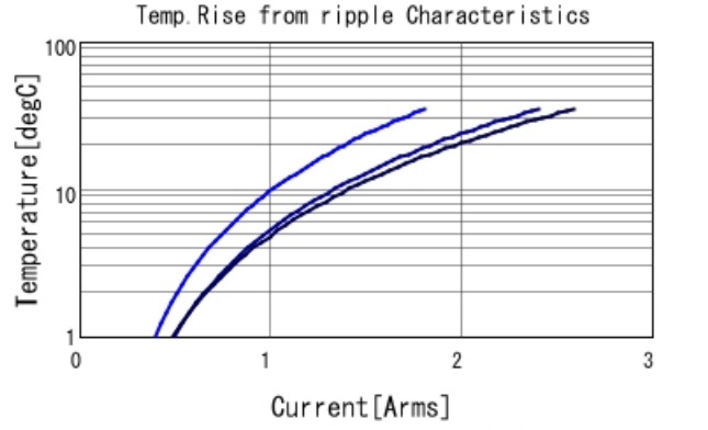
GCJ21BR71H334MA12 Temp. rise — 300kHz — 600
