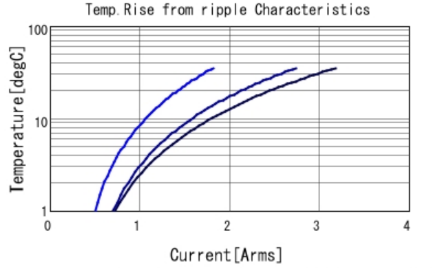
GCJ21BL8YA474KA01 Temp. rise — 200kHz — 500
