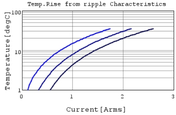
GRT155R61A474KE01 Temp.rise — 100kHz —
