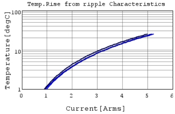
KRM55QR71E336KH01 Temp.rise 50kHz
