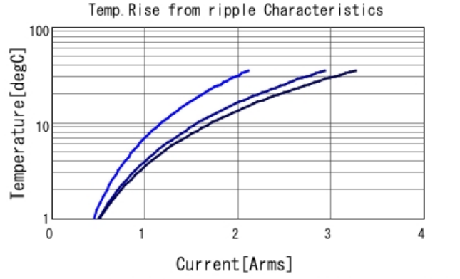
GCJ21BR71C684MA01 Temp. rise — 200kHz — 500
