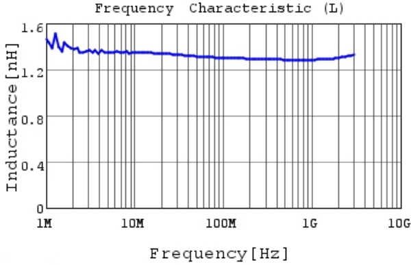
LQW15AN1N3C8Z L
