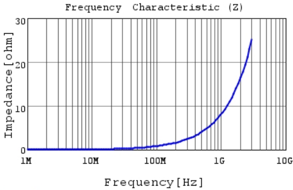
LQW15AN1N3C8Z |Z|
