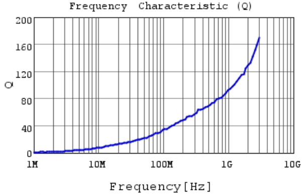
LQW15AN1N3C8Z Q
