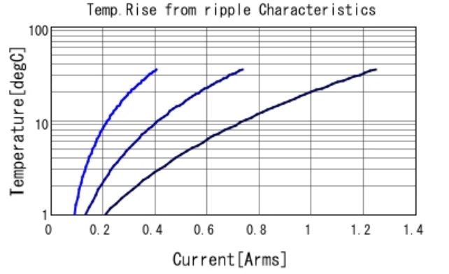
GR331AD72E333KW01 Temp. rise — 30kHz — 100kHz
