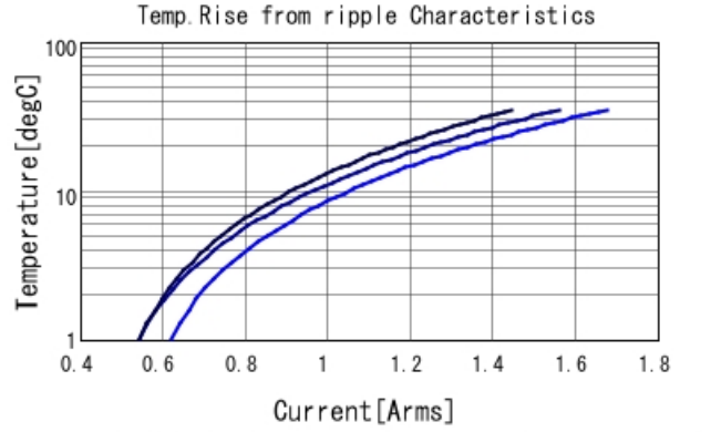
GQM2195G2E360JB12 Temp. rise — 500MHz — 700I
