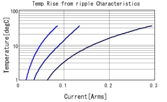
GRM31BR73A472KW01 Temp. rise — 30kHz — 100kHz
