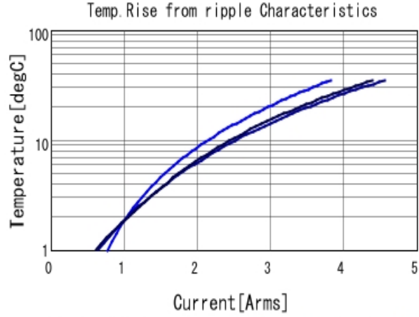
GJ431CC81E105KA01 Temp. rise ■ 100kHz ■ 500kHz ■ 1MHz
