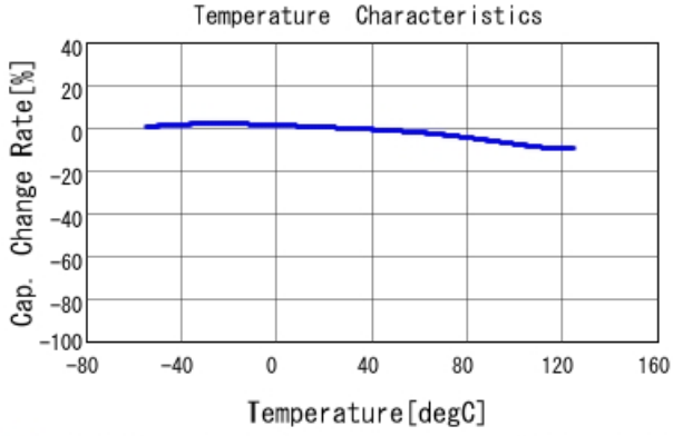
■ GRM21BR72A474MA73 C-Temp. capchange, DCO. 0V, AC1. 0Vrm
