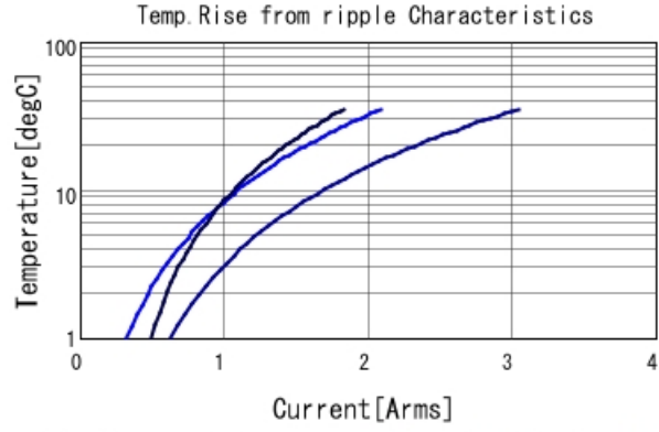
GRM21BR72A474MA73 Temp. rise ■ 200kHz ■ 500kHz ■ 1MHz
