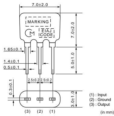
SFVLF10M7LF00-B0
