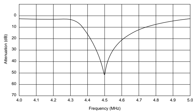
TPSKA4M50B00-R1
