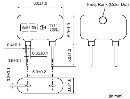
CDALF10M7G_Series
