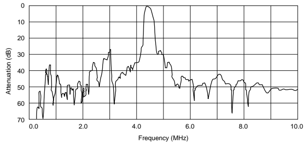
SFSKA4M50CF00-R1
