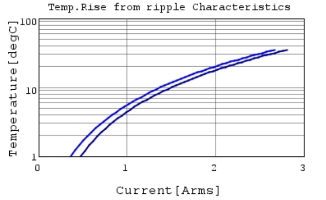
GRM033R60J225ME47 Temp.rise — 500kHz
