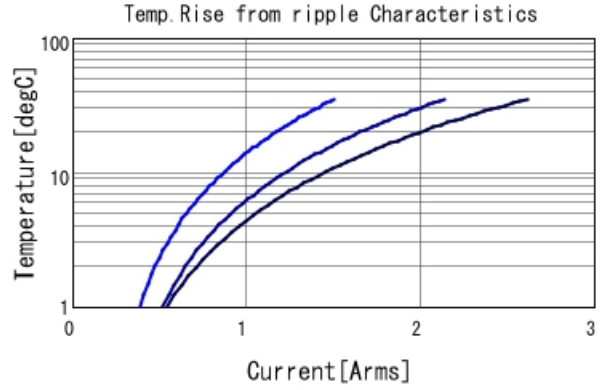
GRM219R71E224MA01 Temp. rise — 300kHz — 600
