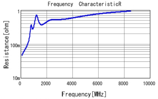
GCM1555G1H561JA16 R DCOV, 25degC
