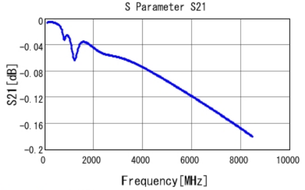
GCM1555G1H561JA16 S21 DCOV, 25degC
