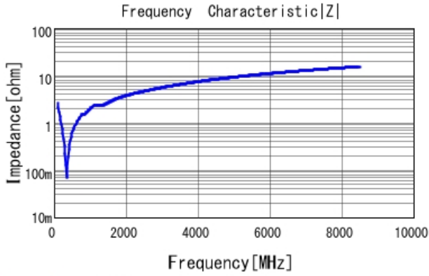
GCM1555G1H561JA16 |Z| DCOV, 25degC
