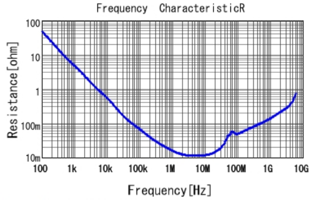
GRM155C81H104KE19 R DCOV, 25degC
