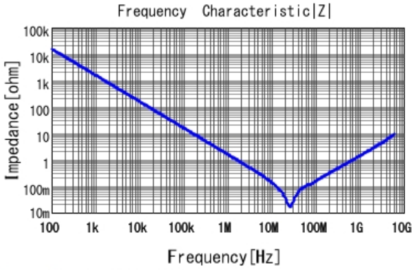
GRM155C81H104KE19 |Z| DCOV, 25degC
