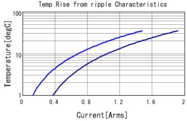
GRM155C81H104KE19 Temp. rise — 500kHz — 1MHz
