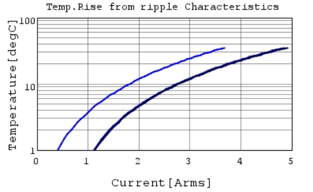
GRM155R60J475ME47 Temp.rise — 100kHz
