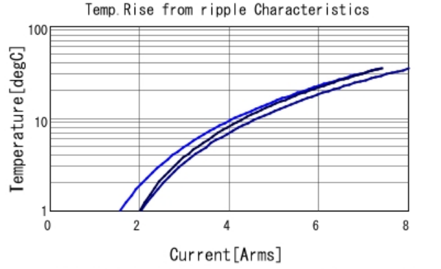
GRM32EB30J107ME16 Temp. rise — 50kHz — 200kHz
