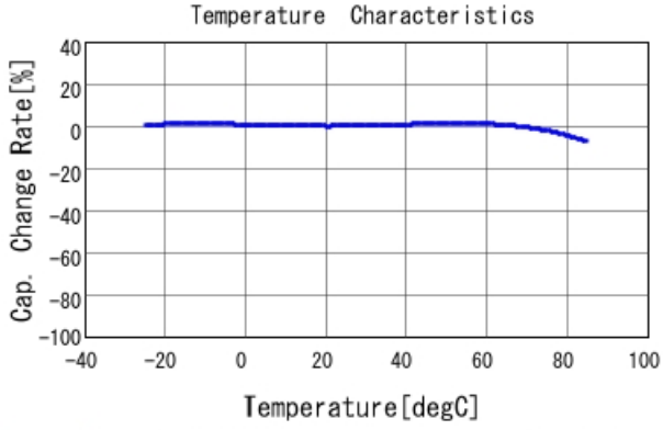
GRM32EB30J107ME16 C-Temp. capchange, DCO. 0V, ACO. 5
