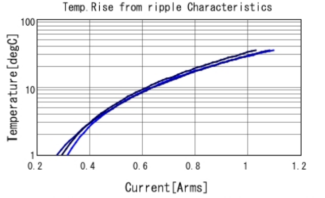
GQM2195C2E5R1DB12 Temp. rise — 700MHz — 1GHz
