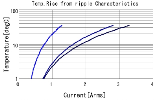
GRM219R71E474MA88 Temp. rise — 100kHz — 500
