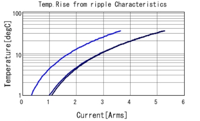
GRM219R61C106MA73 Temp. rise — 80kHz — 400kl
