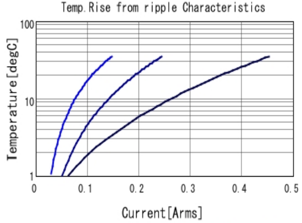
GCJ31CR72J153KXJ3 Temp. rise ■ 30kHz ■ 100kHz ■ 300kHz
