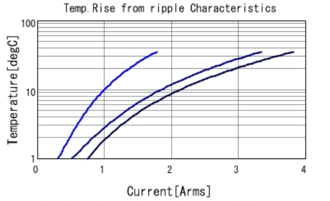
GRM188B10J105KA01 Temp. rise — 100kHz — 500
