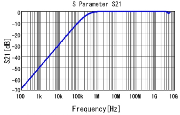
■ GCD188R71H562MA01 S21 DCOV, 25degC
