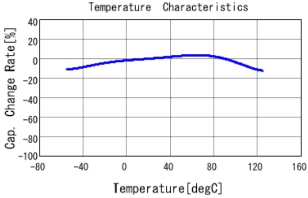
■ GRM21BR71A106MA73 C-Temp. capchange, DCO. 0V, ACO. 35Vr
