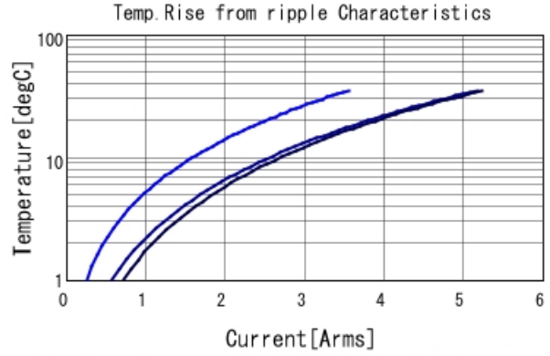
GRM21BR71A106MA73 Temp. rise ■ 80kHz ■ 400kHz ■ 800kHz
