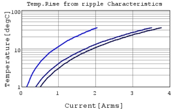
GCM21BR71E225KA73 Temp.rise — 100kHz —
