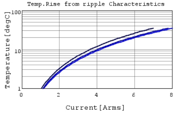
GRM32EC80E227ME05 Temp.rise 50kHz
