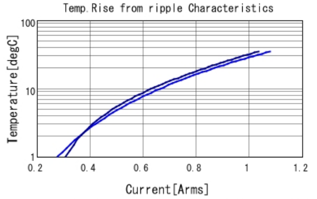
GQM1875C2E2R0CB12 Temp. rise — 2GHz — 3GHz
