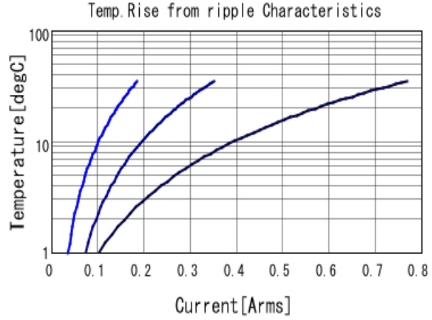
GRJ32DR73A223KWJ1 Temp. rise ■ 30kHz ■ 100kHz ■ 300kHz
