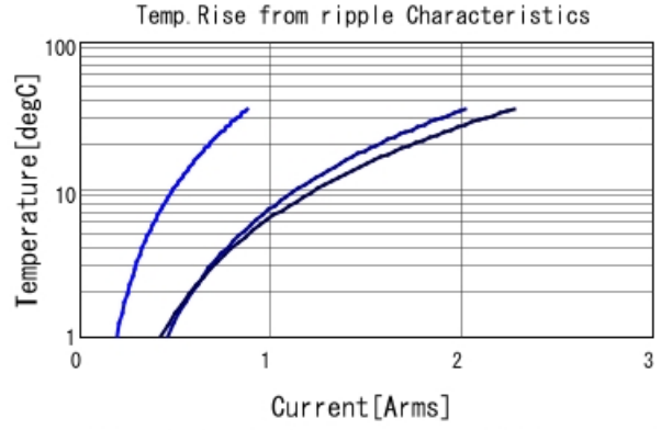
GRM21BR71H224KA01 Temp. rise — 100kHz — 500
