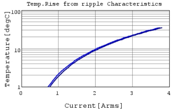
GRT188R61H225KE13 Temp.rise — 500kHz
