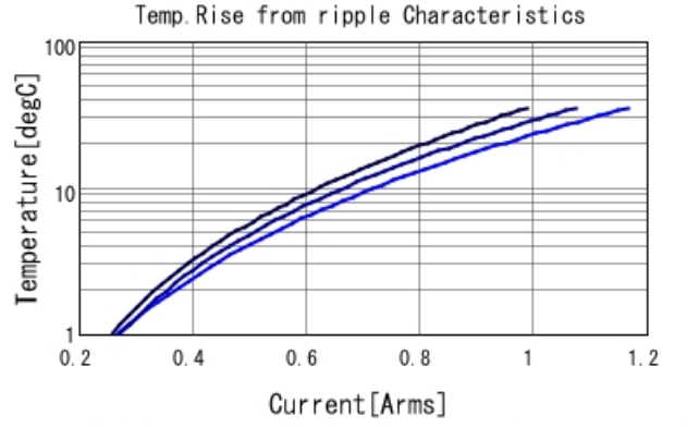
GRM1555C1H150GA01 Temp. rise — 500MHz — 700I
