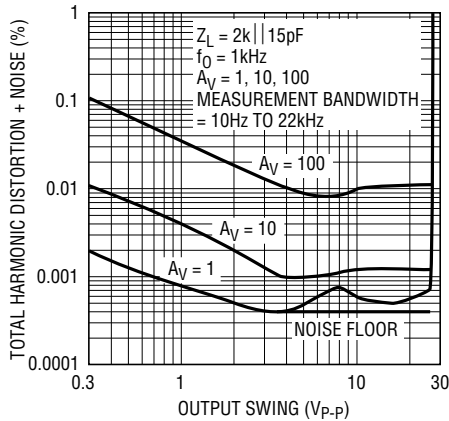
LT1169 • TPC25
