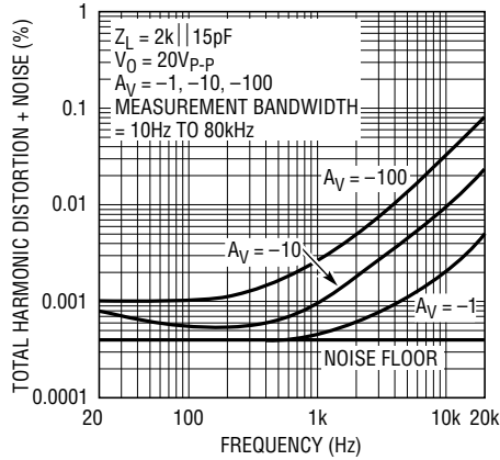
LT1169 • TPC23
