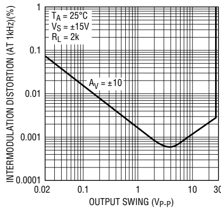
LT1169 • TPC26
