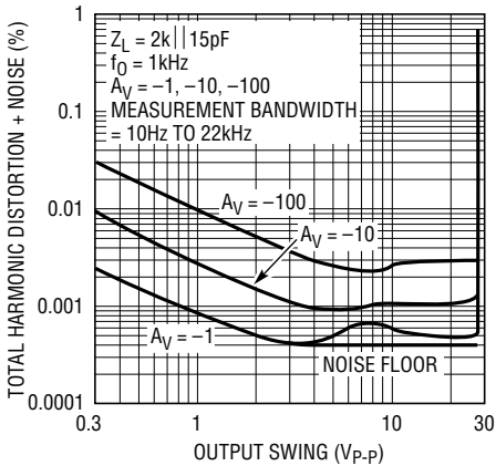
LT1169 • TPC24
