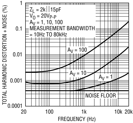
LT1169 • TPC22
