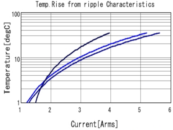
GRJ32EC71H106ME11 Temp. rise ■ 80kHz ■ 400kHz ■ 800kHz
