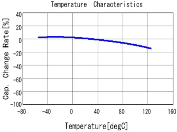
■ GRJ32EC71H106ME11 C-Temp. capchange, DCO. 0V, AC1.0V rm
