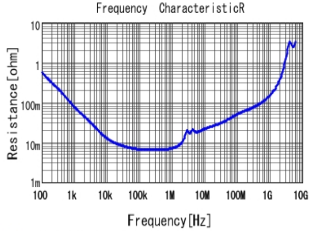
■ GRJ32EC71H106ME11 R DCOV, 25degC
