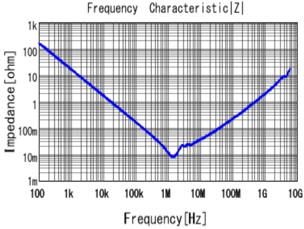
■ GRJ32EC71H106ME11 |Z| DCOV, 25degC
