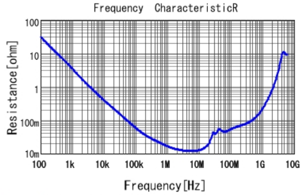
GRM21BR71E224KA01 R DCOV, 25degC
