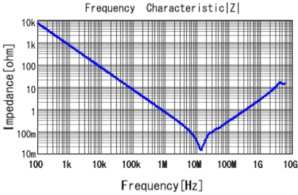
GRM21BR71E224KA01 |Z| DCOV, 25degC
