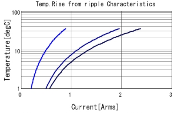
GRM21BR71E224KA01 Temp. rise — 100kHz — 500
