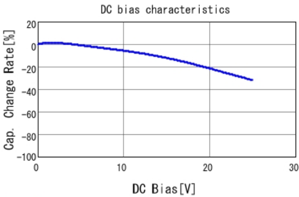
GRM21BR71E224KA01 C-DC bias capchange, 25.0degC, A
