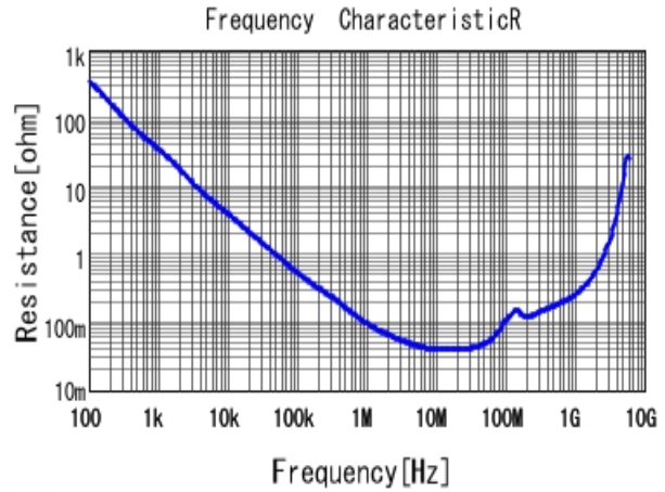
■ GCE188R71E273KA01 R DCOV, 25degC
