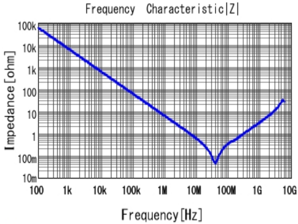
■ GCE188R71E273KA01 |Z| DCOV, 25degC
