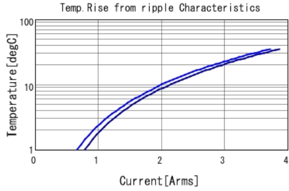
GRM188C81E225KE11 Temp. rise ■ 500kHz ■ 1MHz
