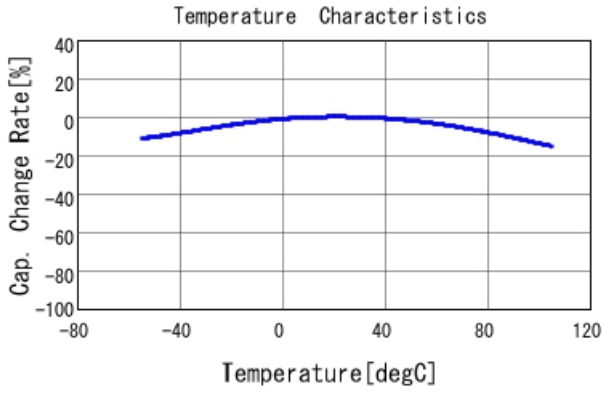
■ GRM188C81E225KE11 C-Temp. capchange, DCO. 0V, ACO. 5Vrm
