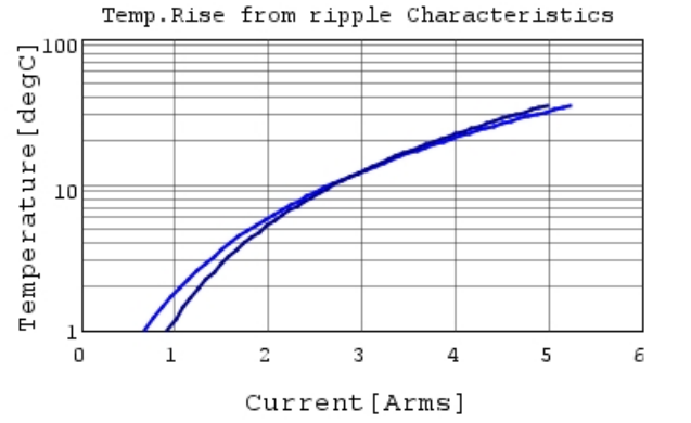
GRM219R6YA475MA73 Temp.rise — 500kHz
