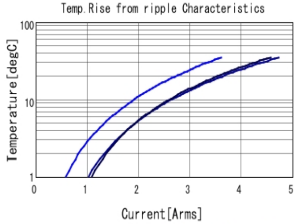
GRJ31CR71E106KE11 Temp. rise ■ 80kHz ■ 400kHz ■ 800kHz
