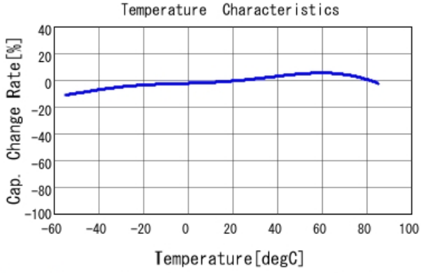
GRM32ER60J476KE64 C-Temp. capchange, DCO. 0V, ACO. 5
