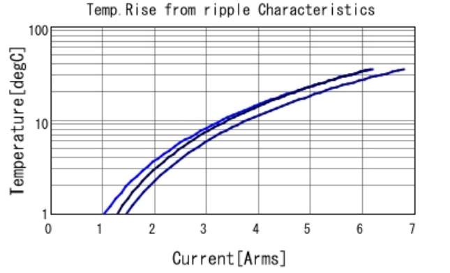
GRM32ER60J476KE64 Temp. rise — 60kHz — 300kHz
