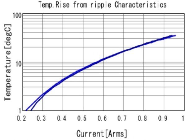
■ GQM2195C2E1R5BB12 Temp. rise ■ 2GHz ■ 3GHz
