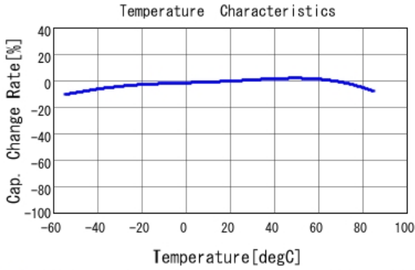
■ GRM187R60J226ME15 C-Temp. capchange, DCO. 0V, ACO. 1Vrm
