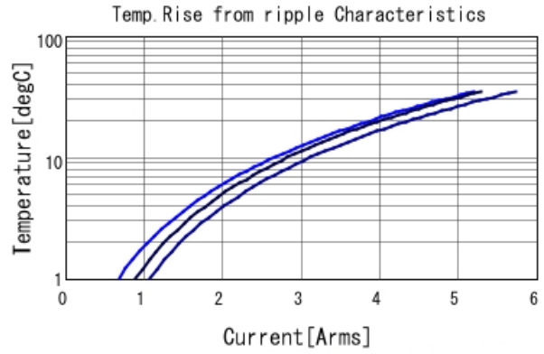
GRM187R60J226ME15 Temp. rise ■ 80kHz ■ 400kHz ■ 800kHz
