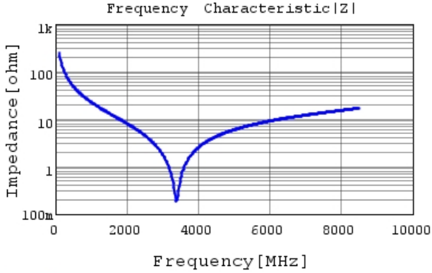
GCQ1555C1H6R4DB01 |Z| DC0V, 25degC
