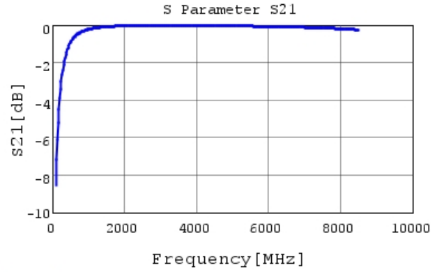
GCQ1555C1H6R4DB01 S21 DCOV, 25degC
