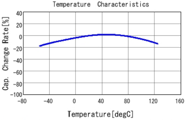
GGM155C71A105KE38 C-Temp. capchange, DCO. 0V, ACO. 2
