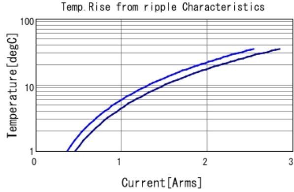
GGM155C71A105KE38 Temp. rise — 500kHz — 1MHz
