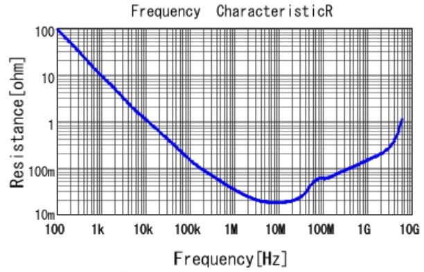
GGM155R71H104KE02 R DCOV, 25degC
