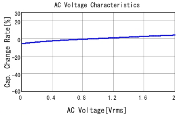
GGM155R71H104KE02 C-AC Voltage capchange, DCOV, 25
