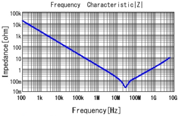
GGM155R71H104KE02 |Z| DCOV, 25degC
