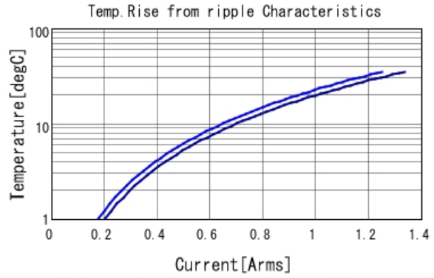
GGM155R71H104KE02 Temp. rise — 800kHz — 1MHz
