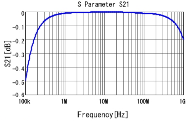
RCER71H473K0A2H03B S21 DCOV, 25degC
