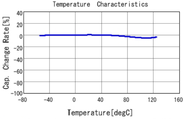
RCER71H473K0A2H03B C-Temp. capchange, DCO. 0V, AC1.
