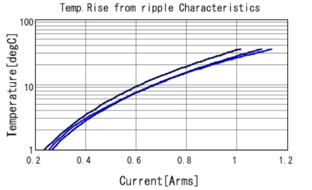
GQM1875C2E150JB12 Temp. rise — 700MHz — 1GHz
