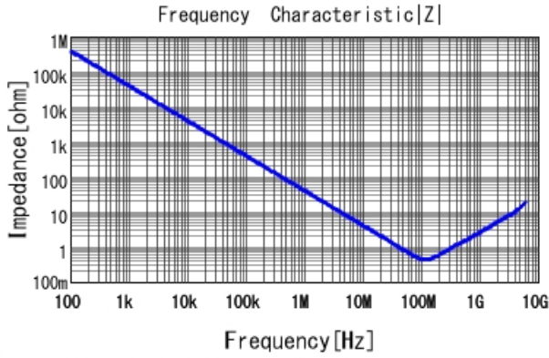
GCJ188R71E392KA01 |Z| DCOV, 25degC
