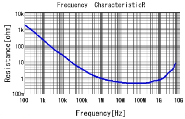
GCJ188R71E392KA01 R DCOV, 25degC
