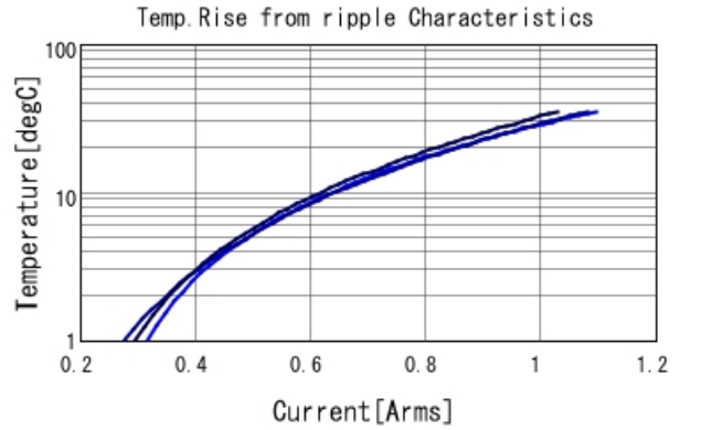
GQM2195G2E5R1CB12 Temp. rise — 700MHz — 1GHz
