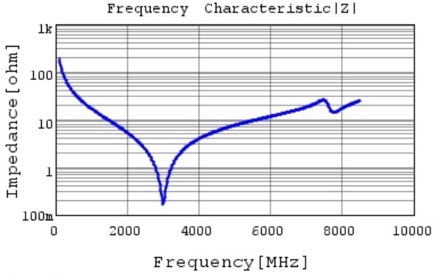
GCQ1555C1H8R4DB01 |Z| DC0V, 25degC
