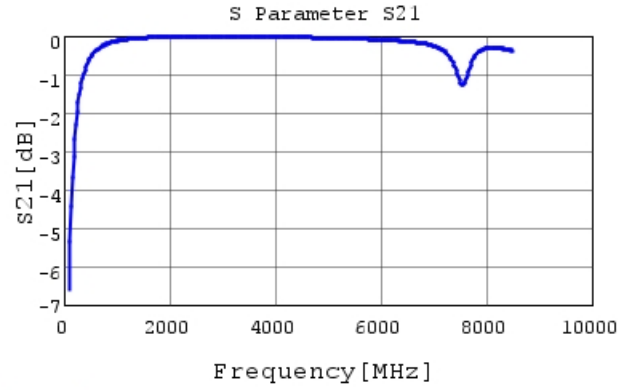
GCQ1555C1H8R4DB01 S21 DCOV, 25degC
